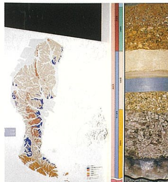
地層の柱状模型
